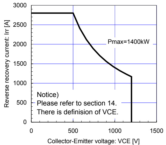
Tj=150°C
