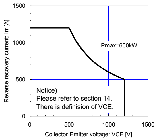
Tj=150°C
